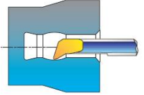
Delik Profil İşleme (MPR)
